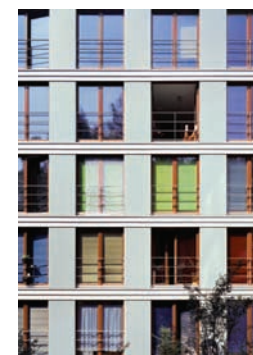
Die neuen, hochgedämmten Fassaden mit den großen französischen Fenstern wurden in vorgefertigten, 12 Meter langen, komplett ausgebauten Holz-Tafelbau-Elementen montiert. Die um ca. 2 m verlängerten Studentenzimmer konnten mit Küche und Bad ausgestattet werden.
