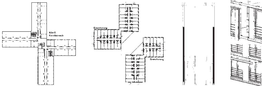
Gebäudegrundriss vorher/nachher: Durch den vorgesetzten Rahmen wurde das Gebäude ausgesteift und der Kernbereich konnte abgerissen werden. Der neu entstandene Platz wird von den verglasten Treppenhäusern gefasst.
